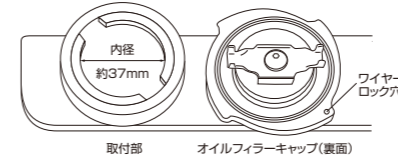
取付部 オイルフィラーキャップ(裏面)
